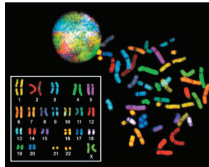
Рис. 30.4. Кариотип людини
