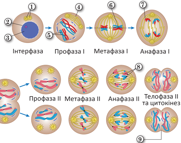
Рис. 31.4. Фази мейозу
