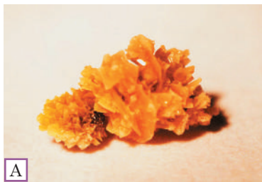
Рис. 24.4. Сечова кислота
